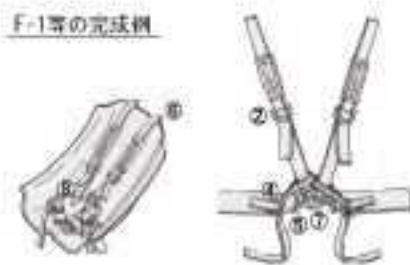
エッチングパーツ部品名
